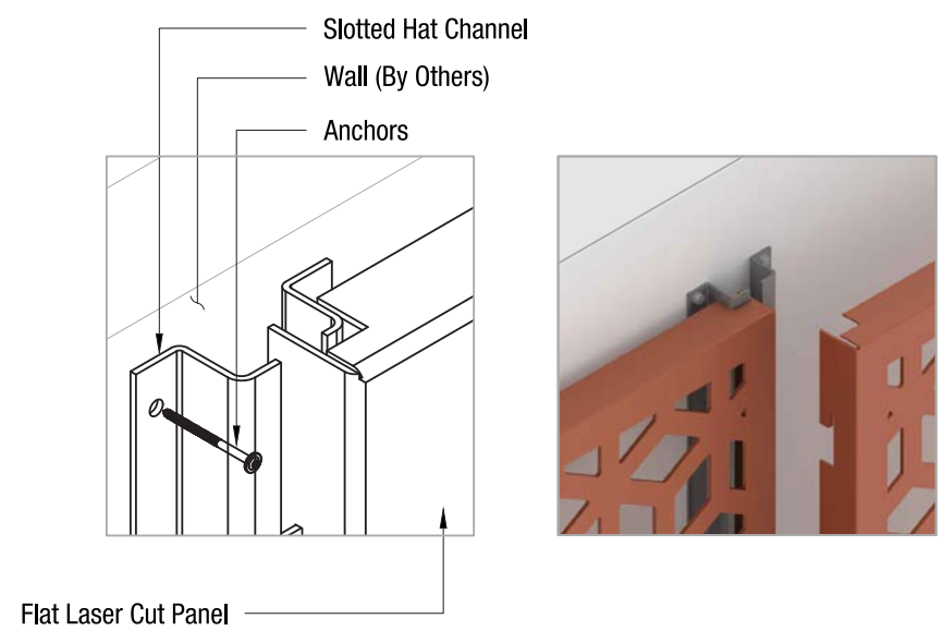
FD1-3 TO CONCRETE/DRYWALL
