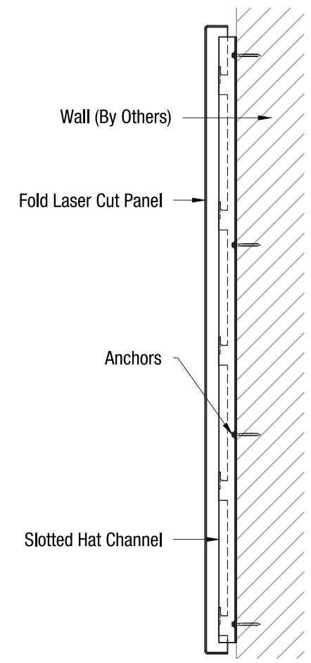
FD1-3 TO CONCRETE/DRYWALL
