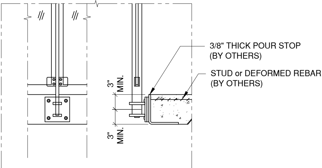
Welded @ Pour Stop - $$ Detail# BE-F05
